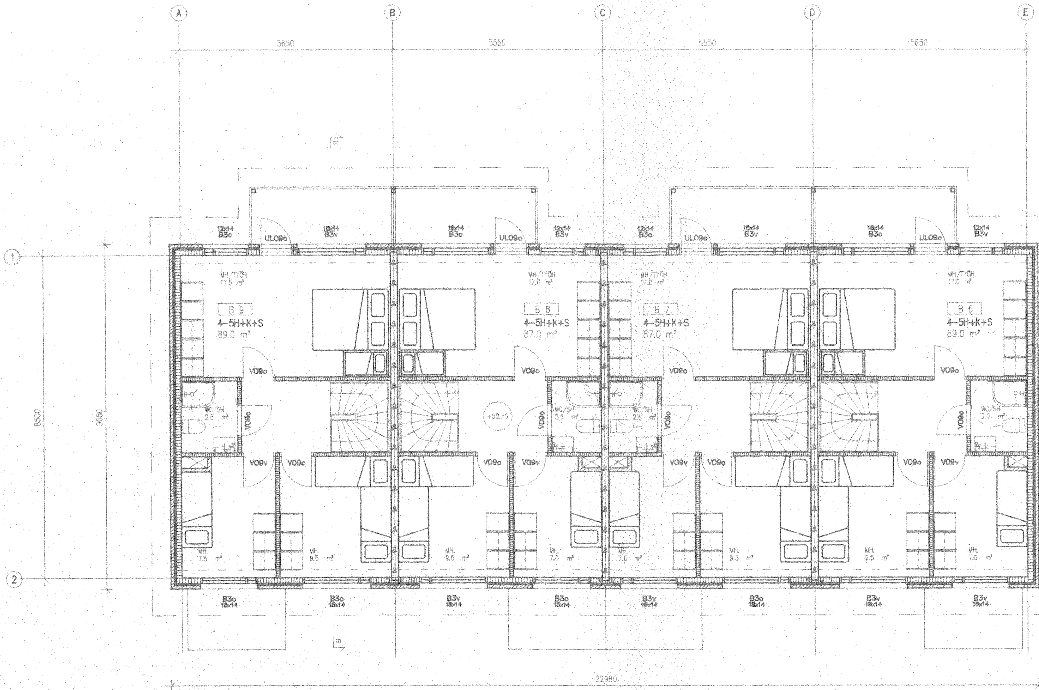
2. KERROS
